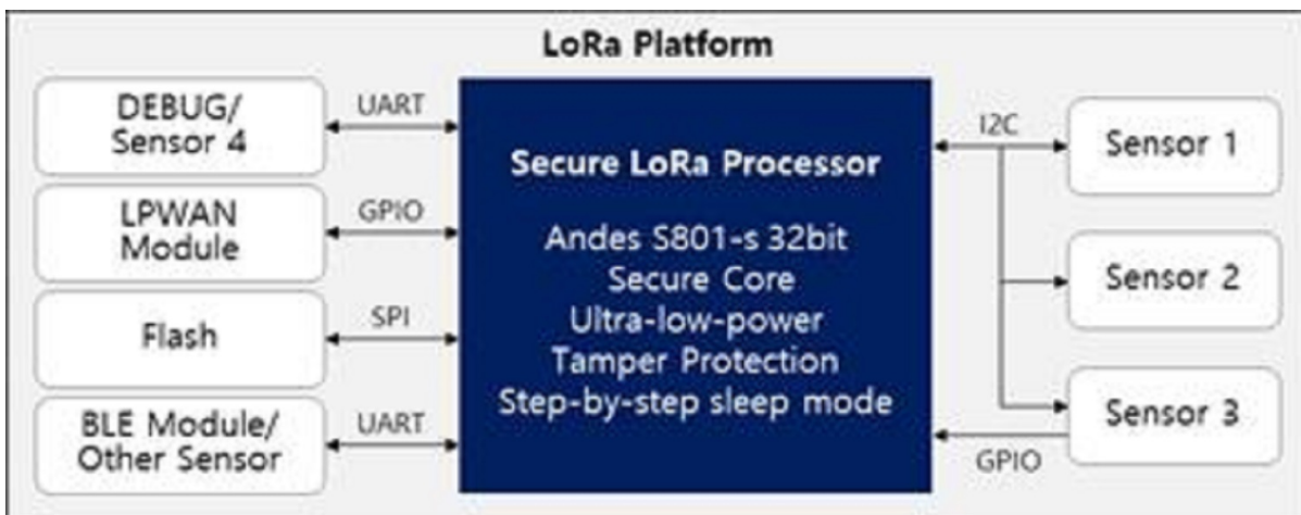
라닉스 LoRa Platform
